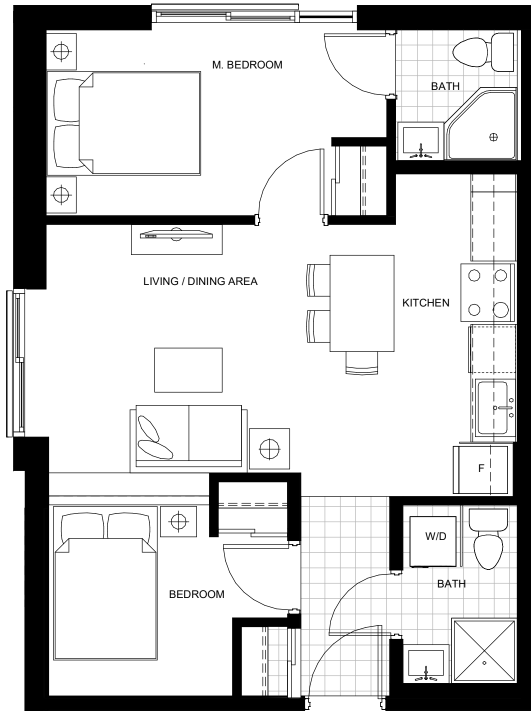
UNIT: 1025
